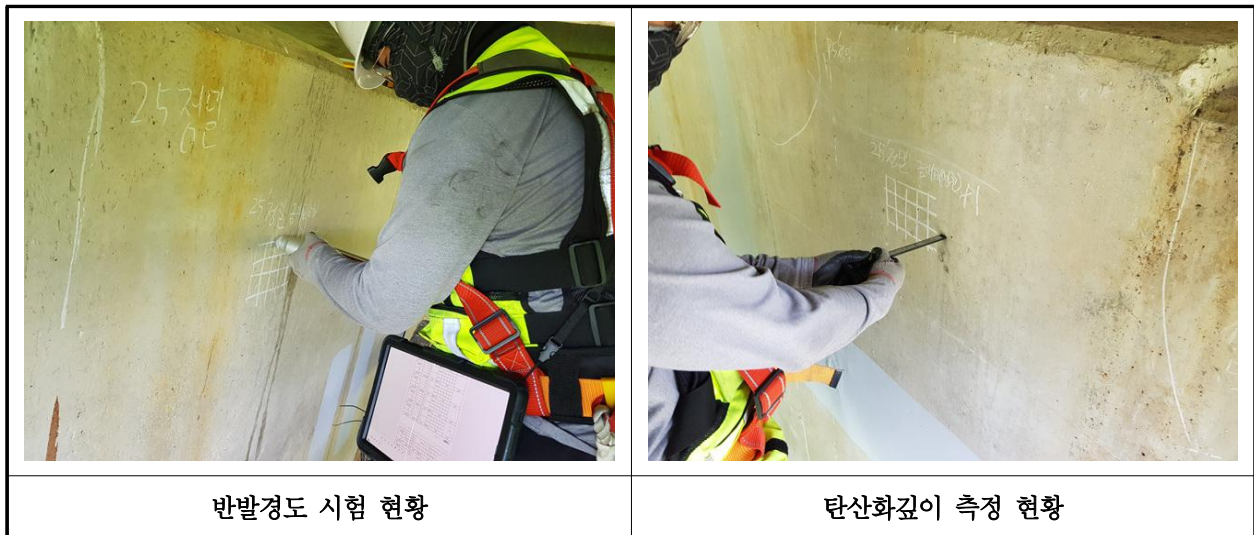
【사진 18.4.1】 콘크리트 내구성조사 현황
