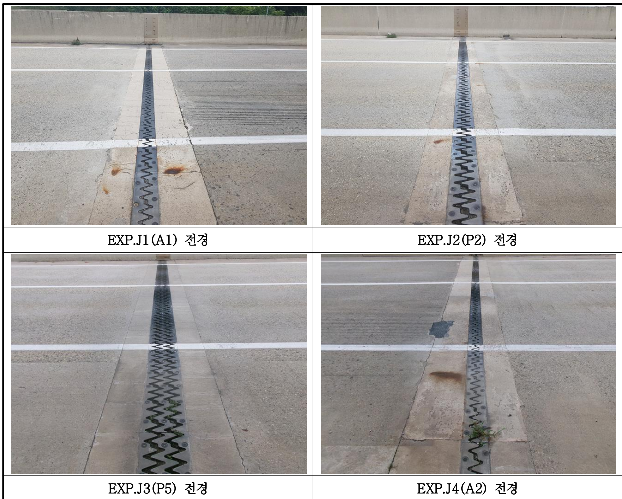
【사진 18.3.17】 신축이음장치 전경
