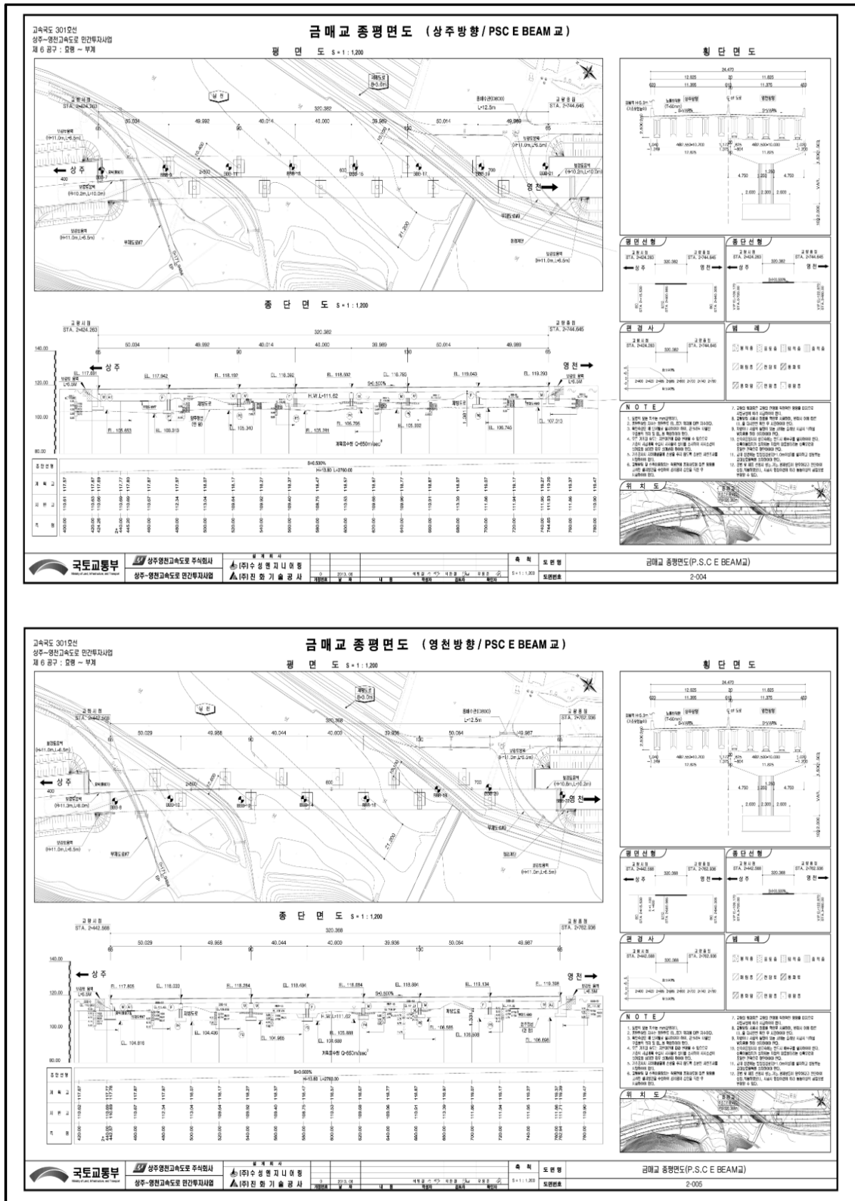
【그림 18.1.3】 종평면도
